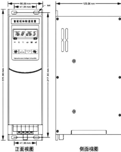
尺寸图
