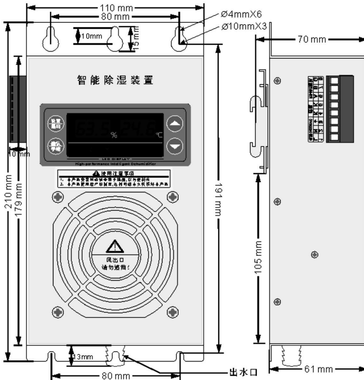
尺寸图
